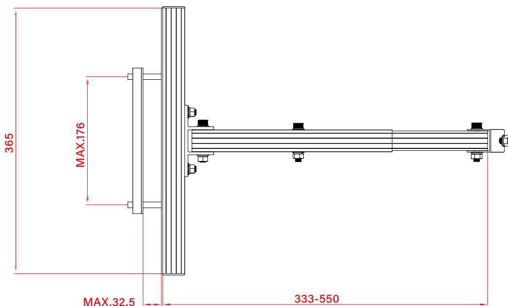
Verstellbarer Träger / Adjustable Bracket
