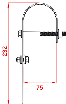
Handlaufhaken / Handrail Hook
